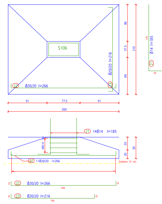
T5 TEMELİ ( 260/ 210 )
